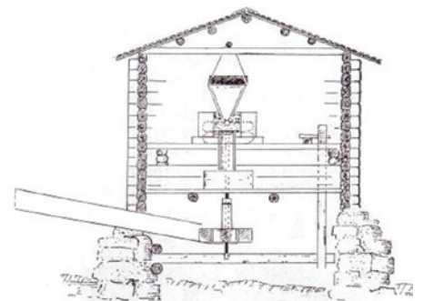
Piirros tyypillisestä jalkamyllystä ja sen jauhatuskoneistosta.
